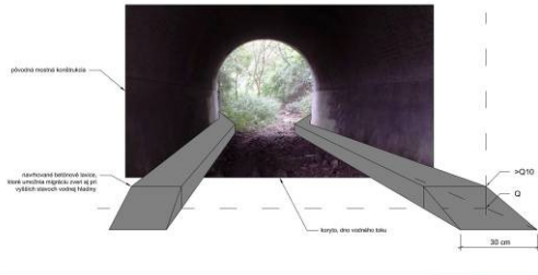
Príloha č. 9: Návrh rekonštrukcie migračného objektu (MO11) na ceste I. triedy (I/51 km 234, Žemberovec)
