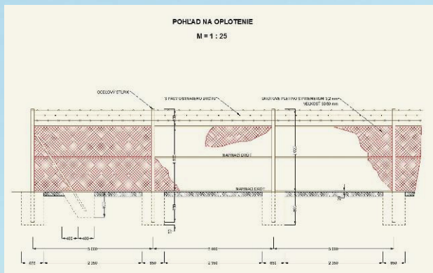
Výkres oplatenia sadu/vinohradu
